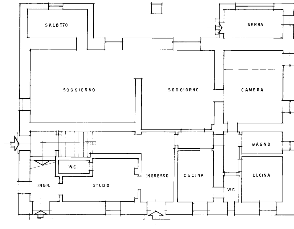
PIANO TERRA h=3.45
