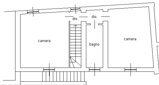
Piano secondo (h. 3.00)
