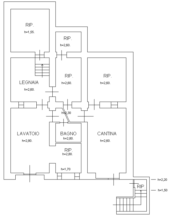
PIANO SOTTOSTRADA
