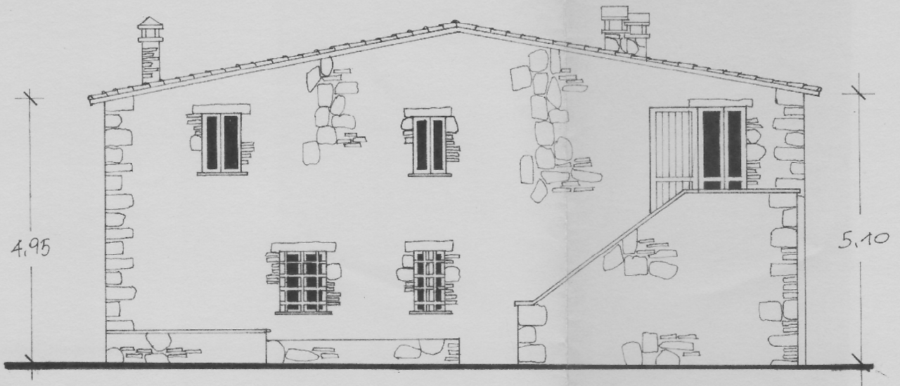
PROSPETTO FRONTALE
