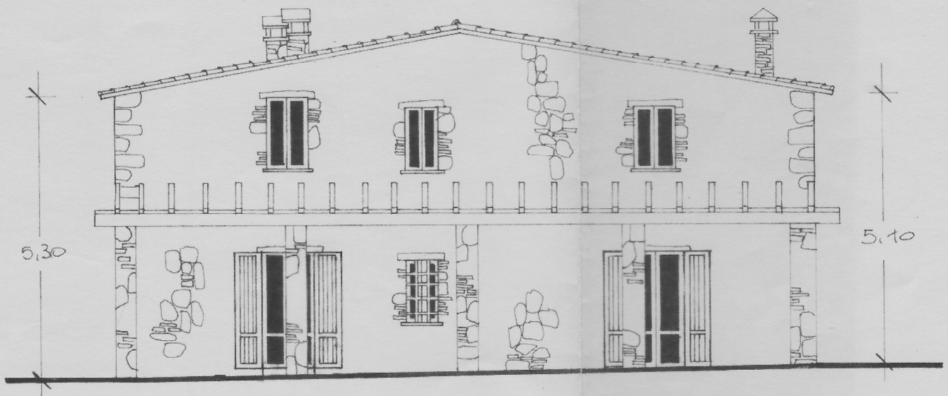
PROSPETTO TERGALE
