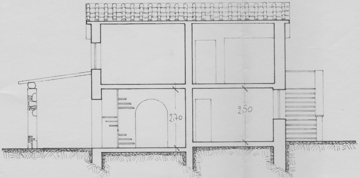
SEZIONE B-B'
