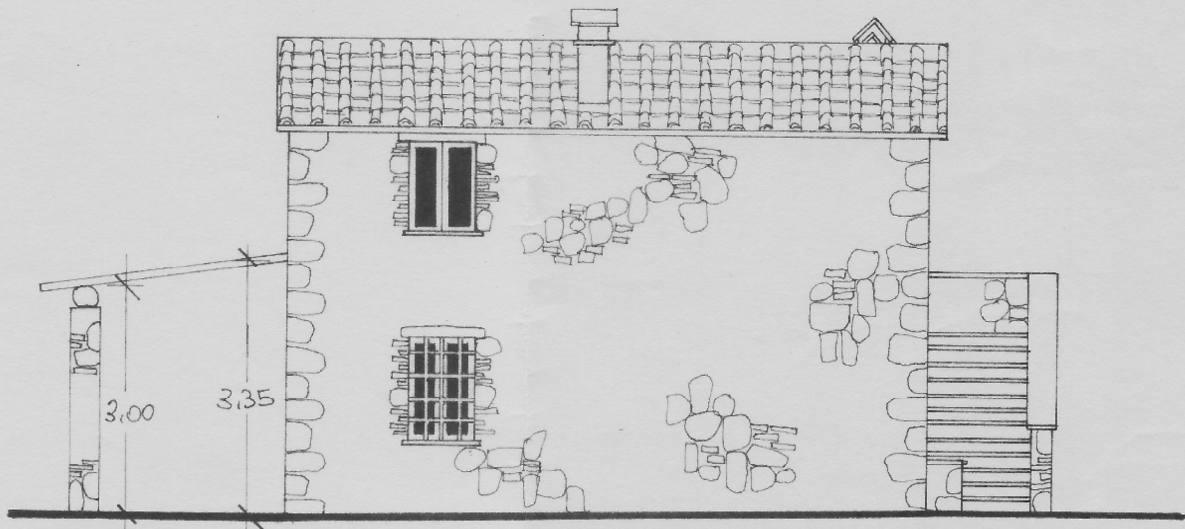
PROSPETTO LATERALE SINISTRO
